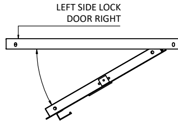
Semi Automatic Swing Door (SDM1-AVC)
