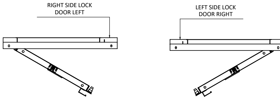
Semi Automatic Swing Door (SDM2-AVC)
